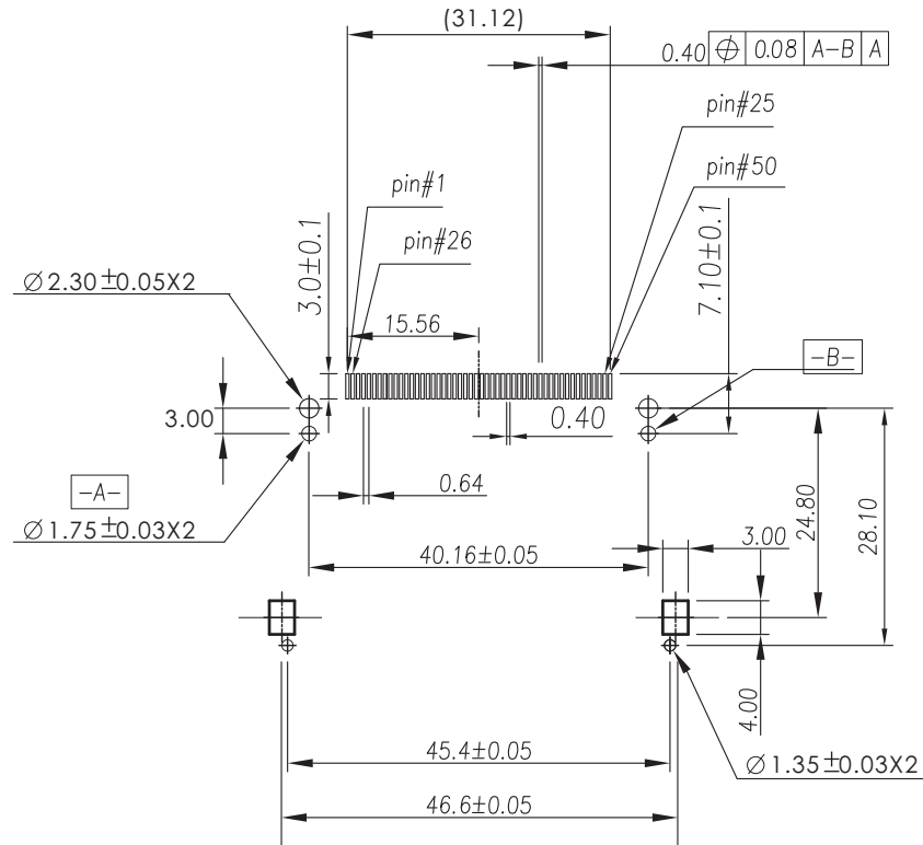
P.C.B Layout
