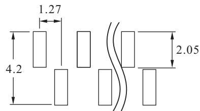
P.C.B Layout A TYPE
