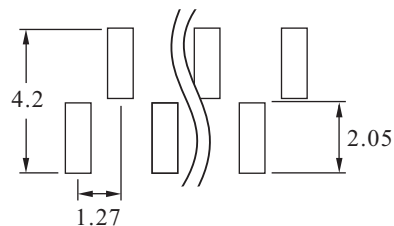
P.C.B Layout B TYPE
