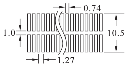
P.C.Board Layout :
