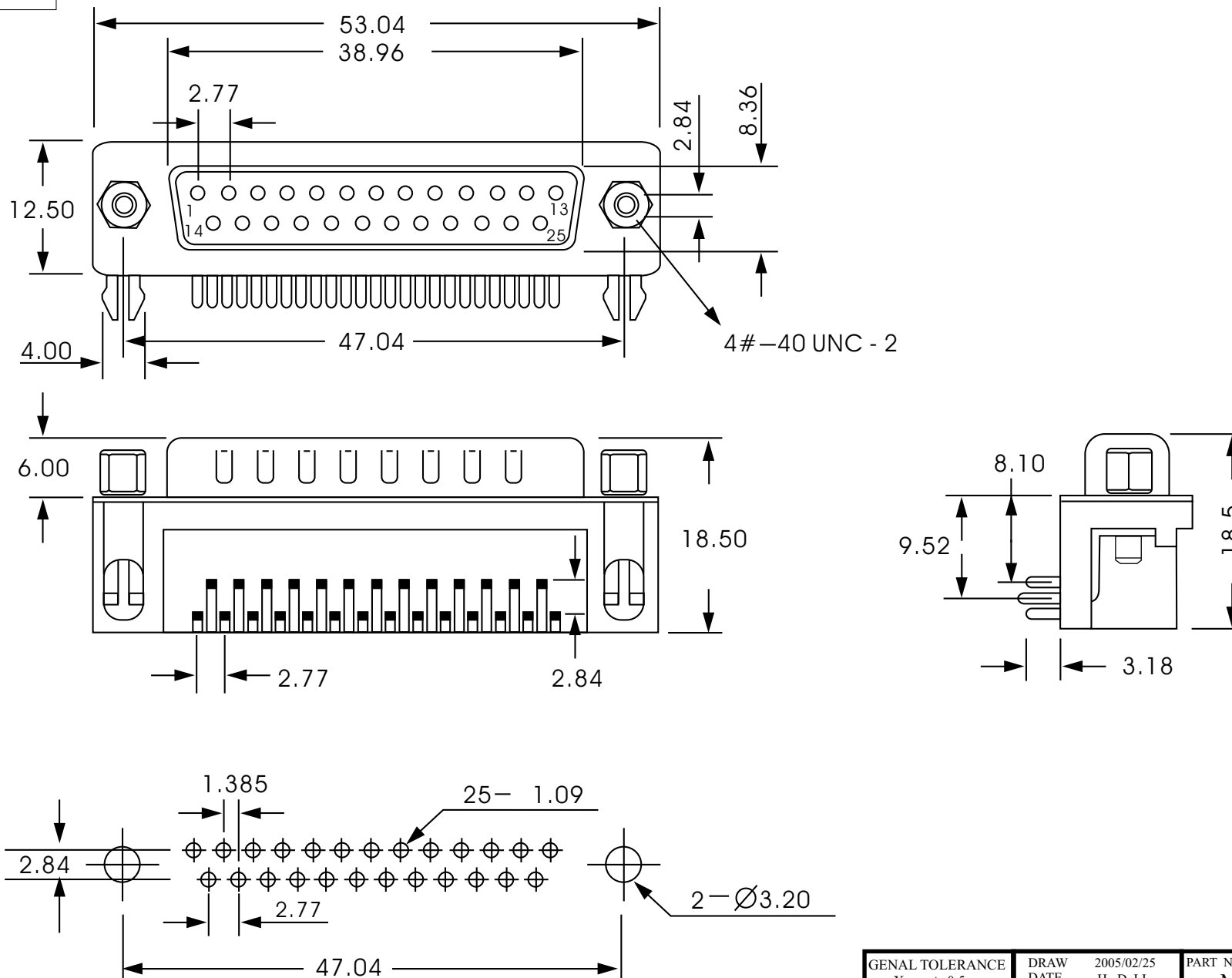
P.C.B LAYOUT
